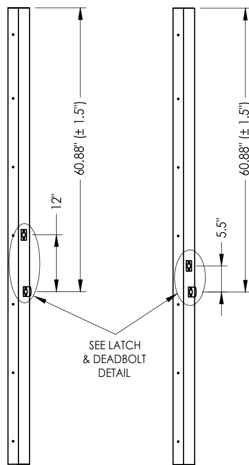
STRIKE JAMB
